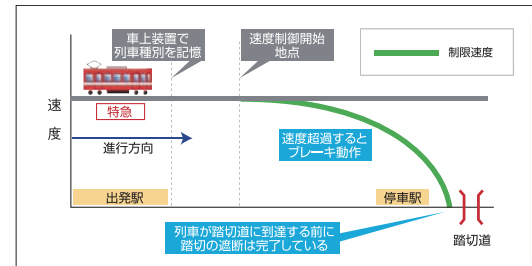
「踏切道防護システム」動作概要
